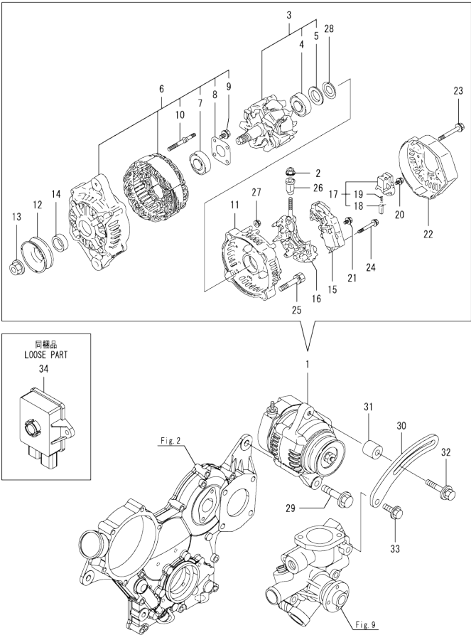
Fig.15. GENERATOR
