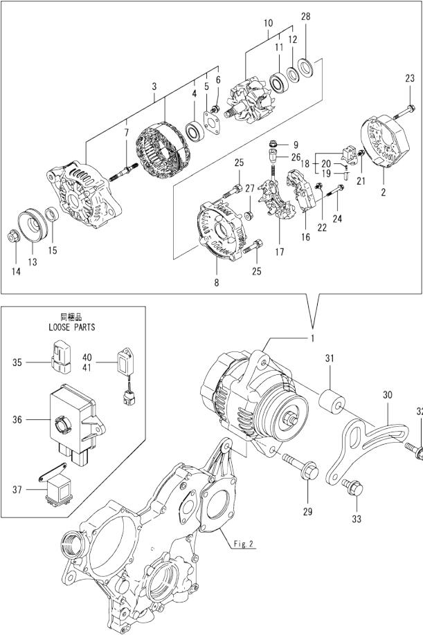
Fig.15. GENERATOR
