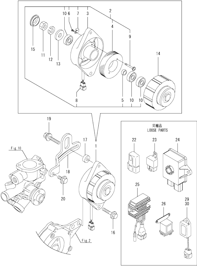
Fig.16. GENERATOR
