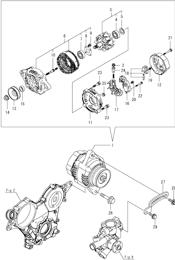
Fig.15. GENERATOR
