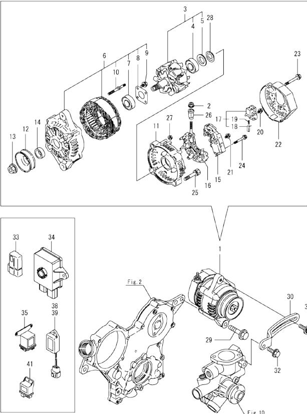
Fig.16. GENERATOR
