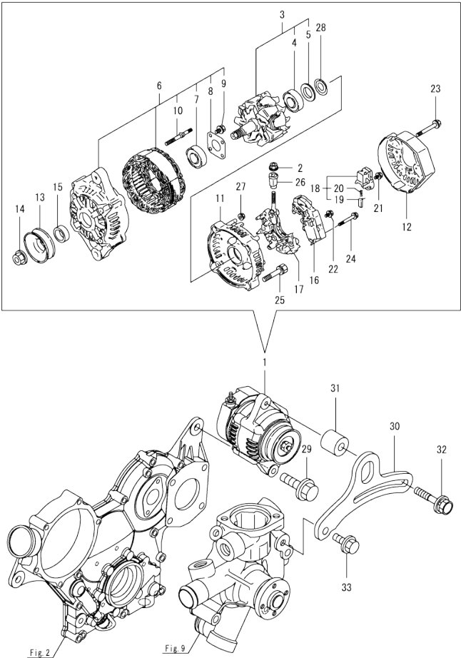
Fig.15. GENERATOR
