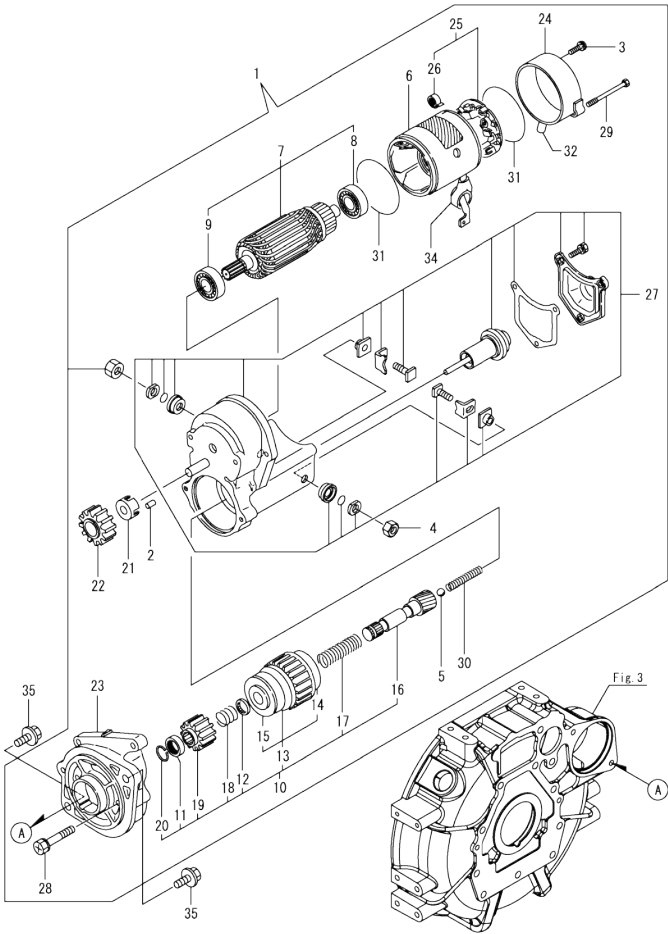
Fig.16. STARTER MOTOR
