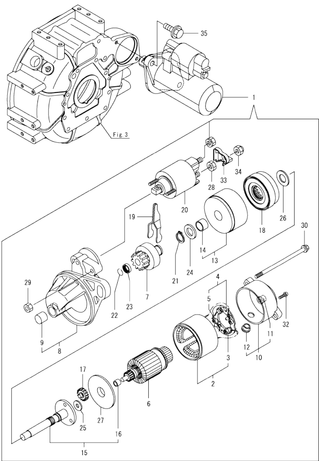
Fig.16. STARTER MOTOR
