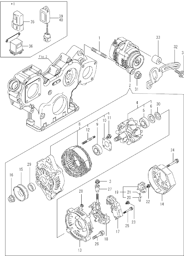
Fig.16. GENERATOR
