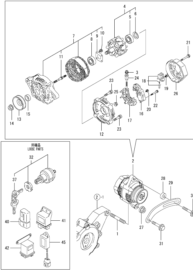
Fig.16. GENERATOR
