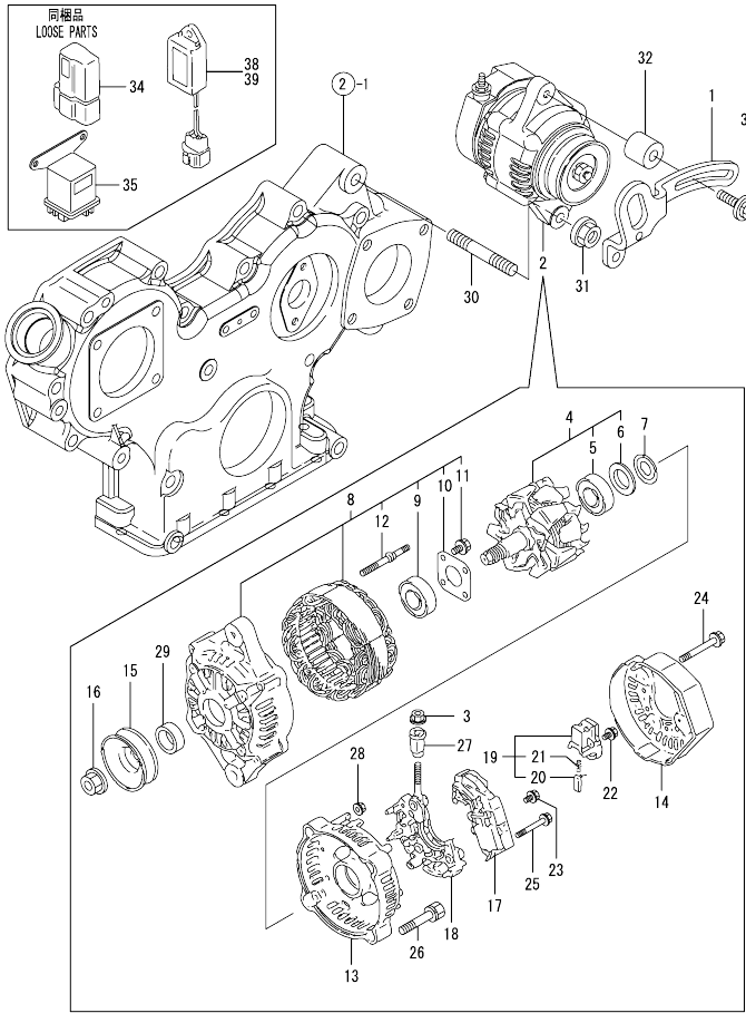
Fig.16. GENERATOR
