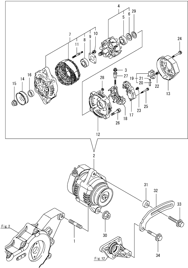
Fig.18. GENERATOR
