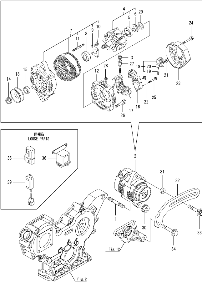
Fig.18. GENERATOR
