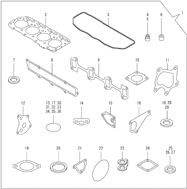
Fig.19. GASKET SET
