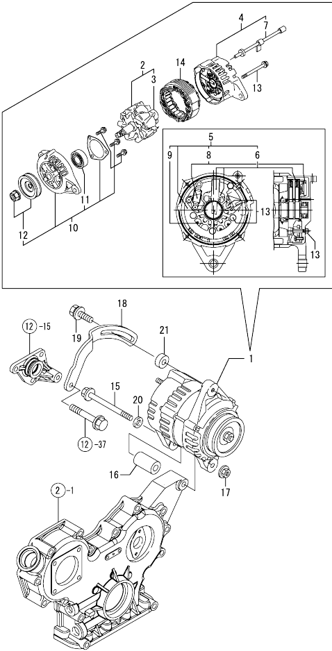
Fig.18. GENERATOR
