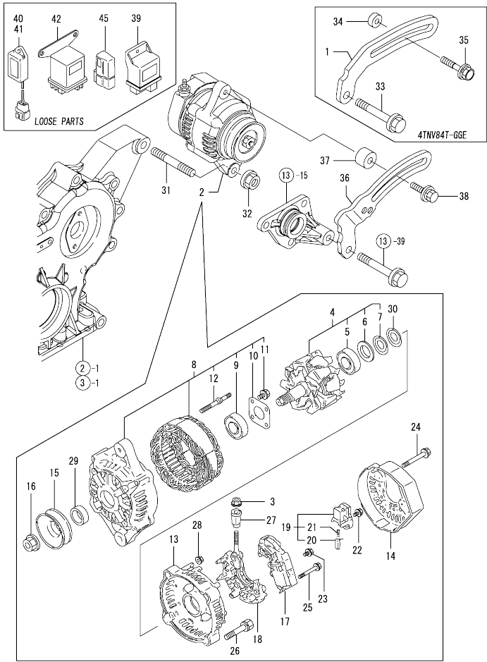
Fig.21. GENERATOR
