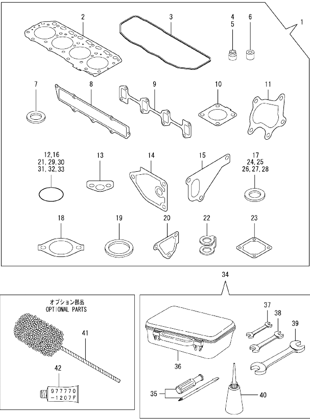
Fig.19. GASKET SET
