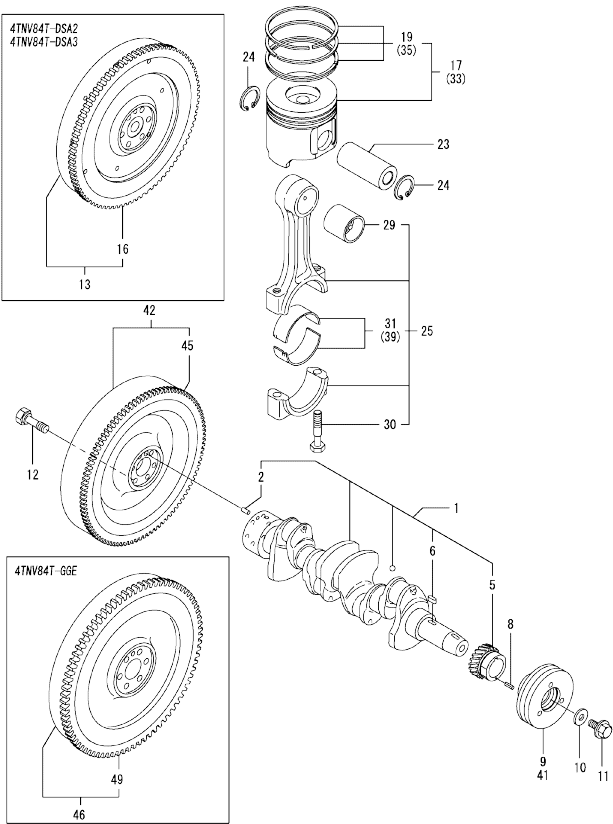
Fig.10. CRANKSHAFT & PISTON
