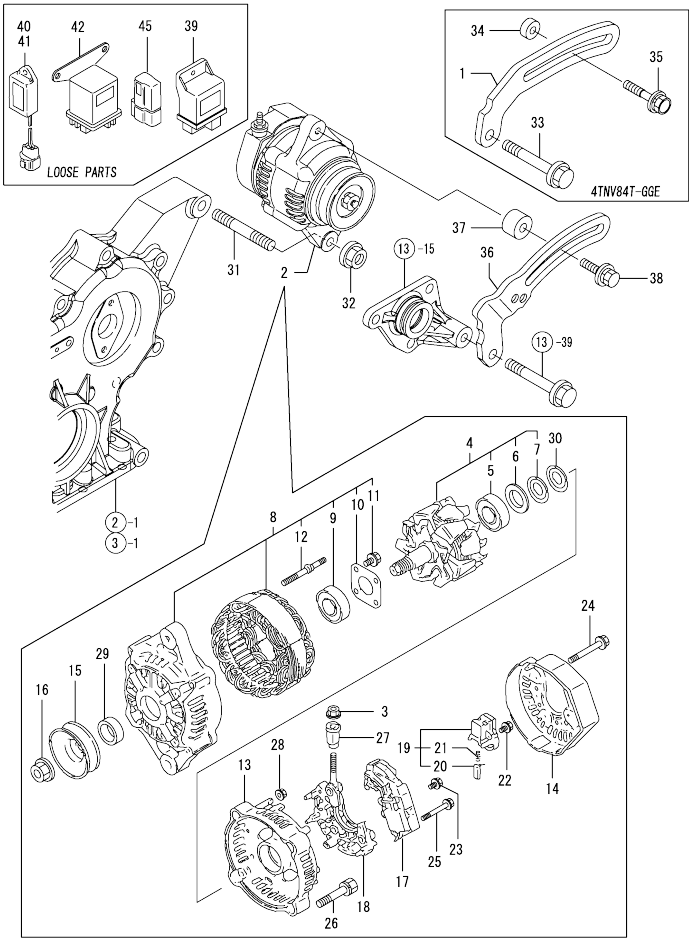
Fig.21. GENERATOR
