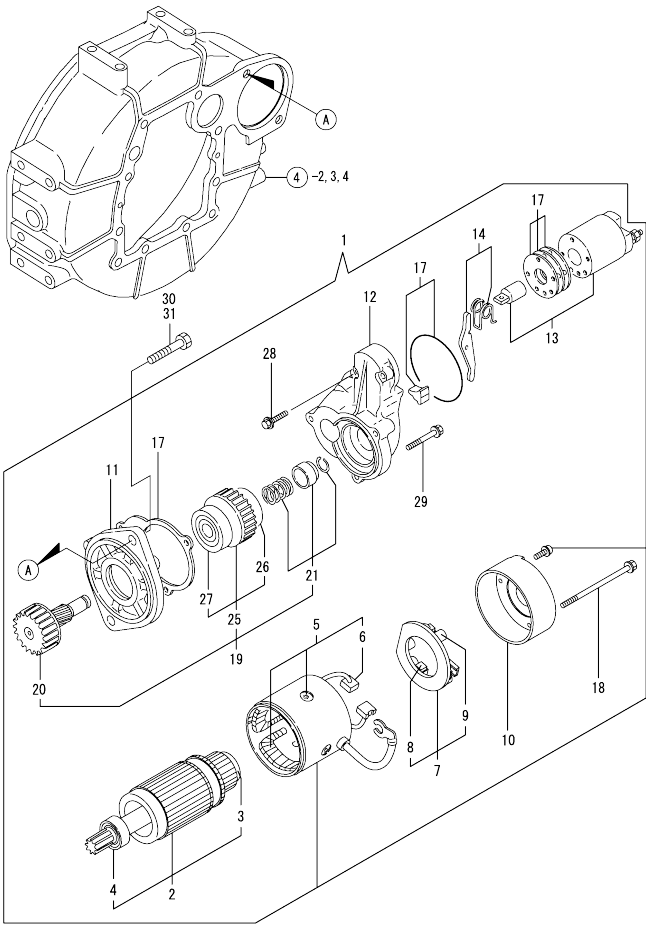
Fig.19. STARTER MOTOR
