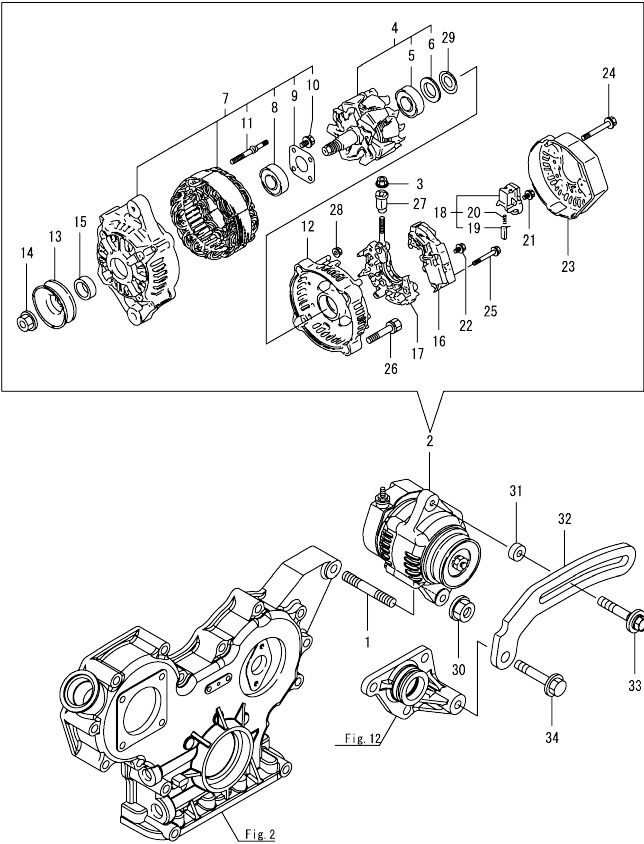
Fig.18. GENERATOR
