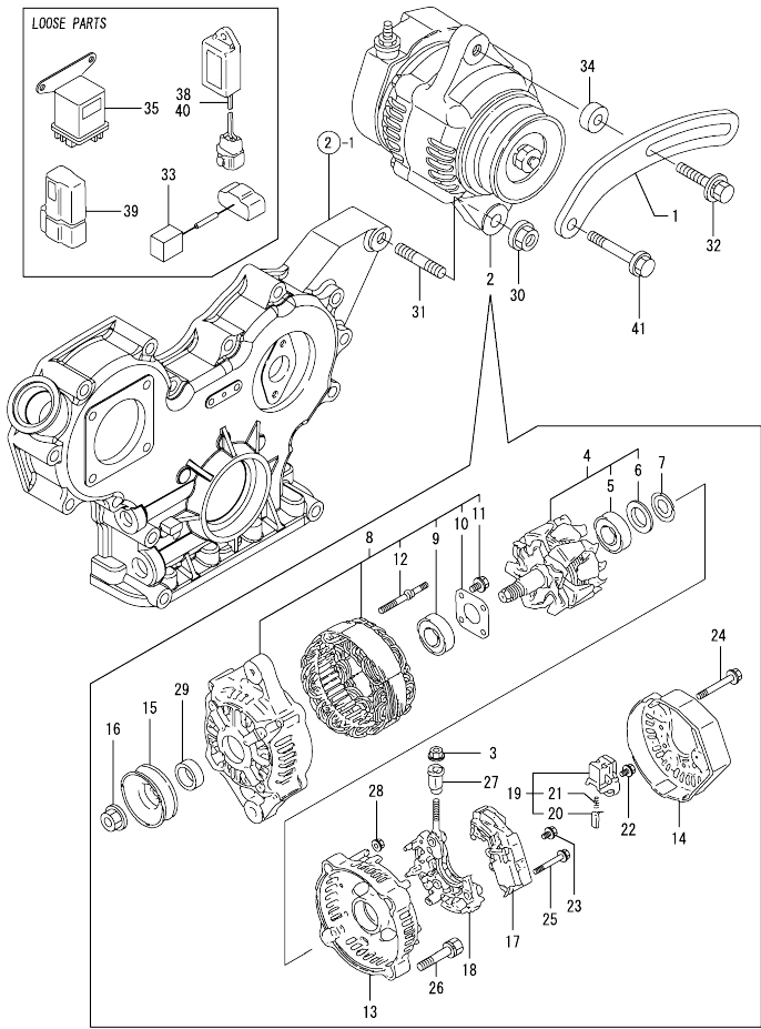
Fig.18. GENERATOR
