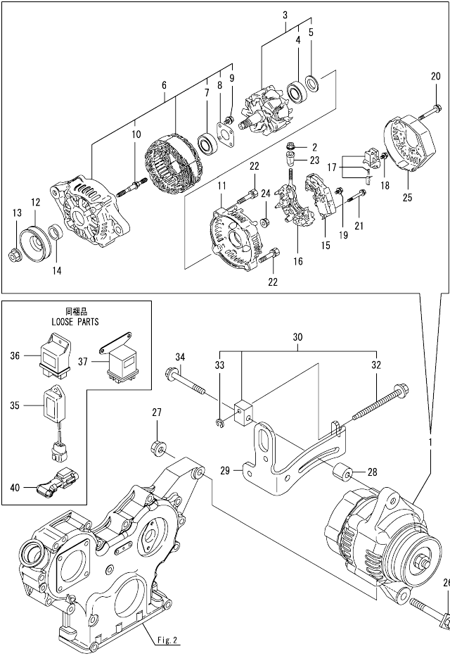
Fig.16. GENERATOR
