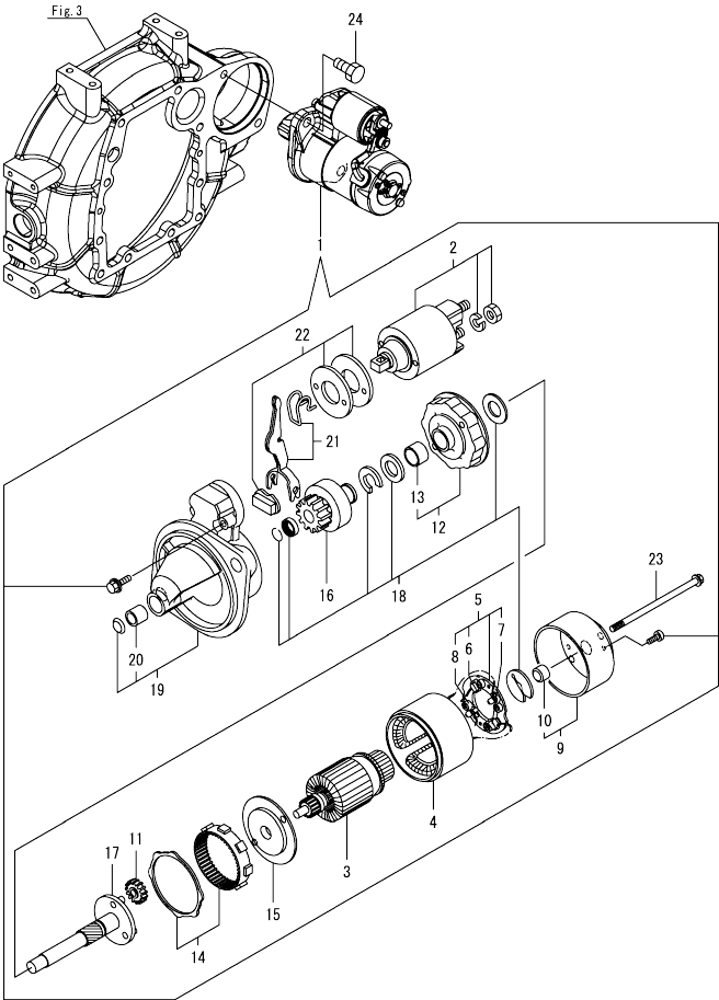
Fig.16. STARTER MOTOR
