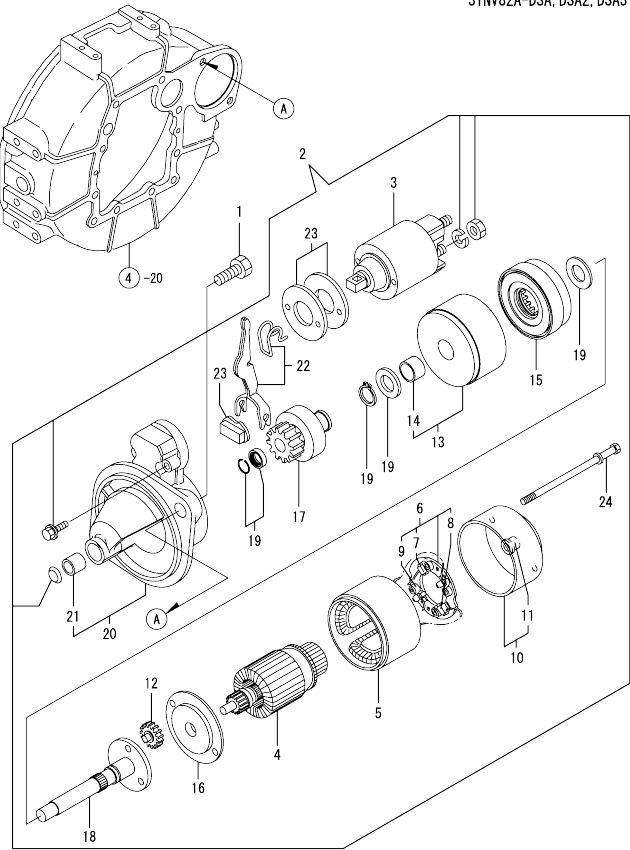
Fig.16. STARTER MOTOR
