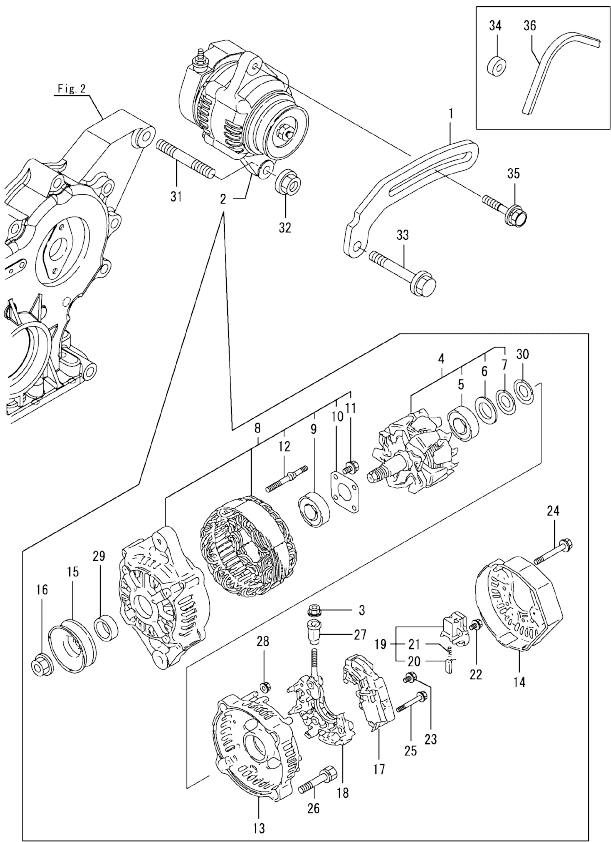
Fig.14. GENERATOR
