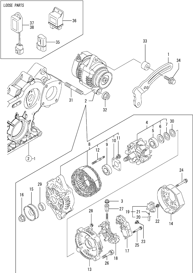
Fig.15. GENERATOR
