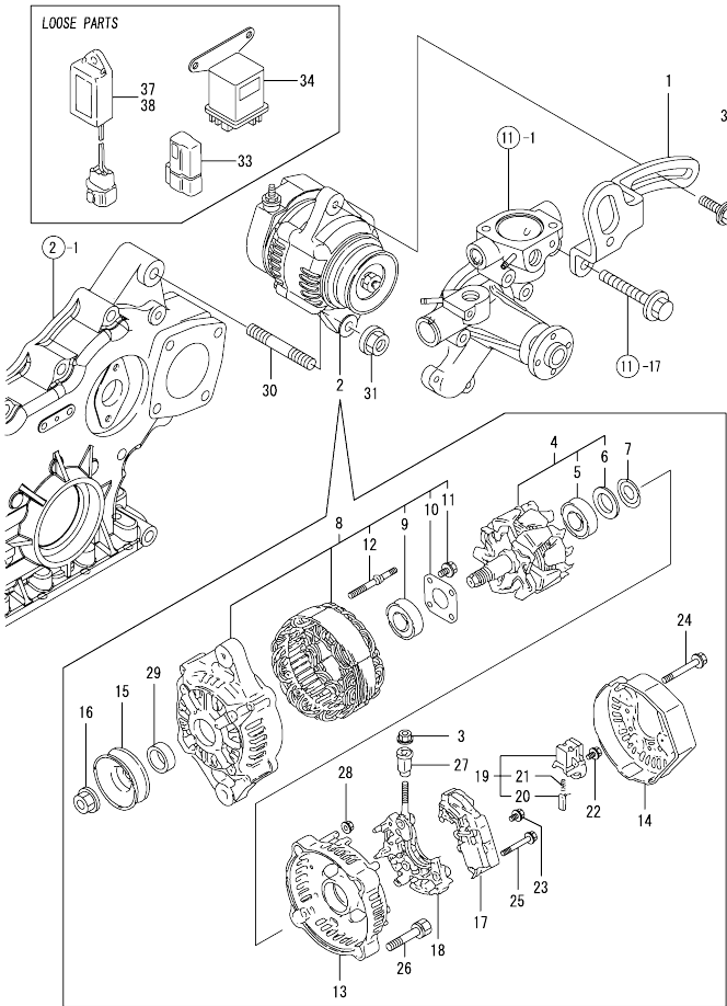
Fig.17. GENERATOR
