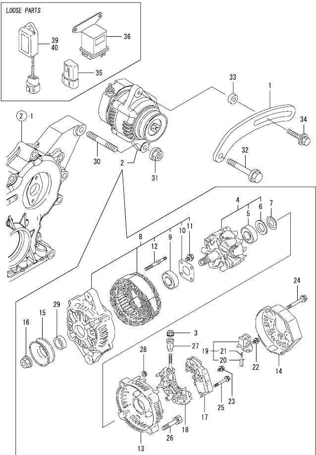
Fig.16. GENERATOR
