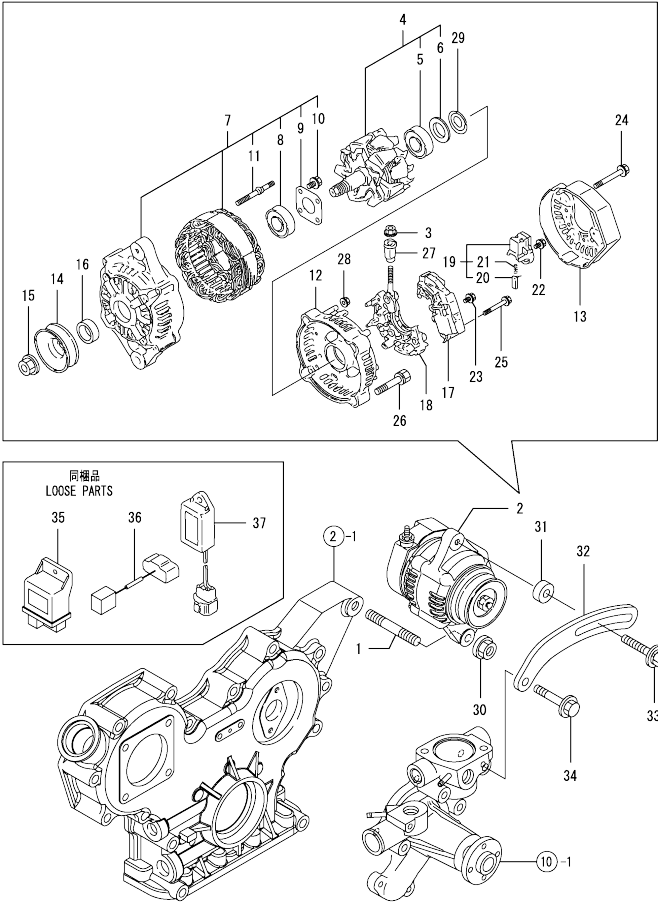
Fig.16. GENERATOR
