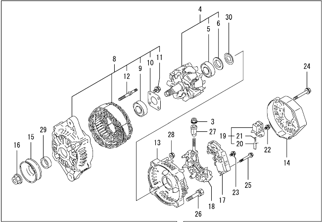
Fig.15. GENERATOR
