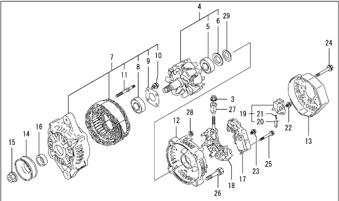
Fig.16. GENERATOR
