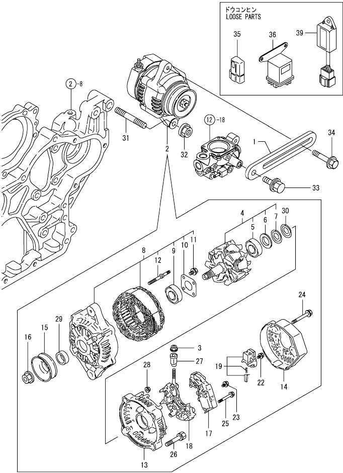
Fig.18. GENERATOR
