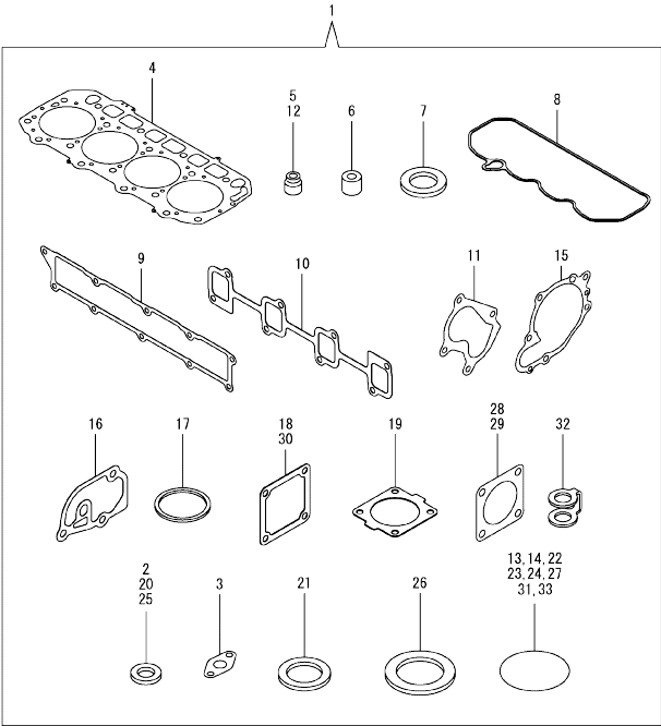
Fig.19. GASKET SET
