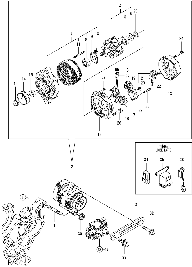
Fig.18. GENERATOR
