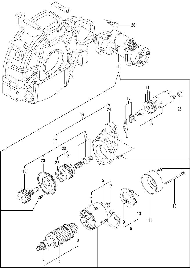
Fig.19. STARTER MOTOR
