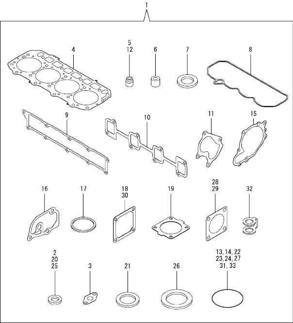
Fig.18. GASKET SET
