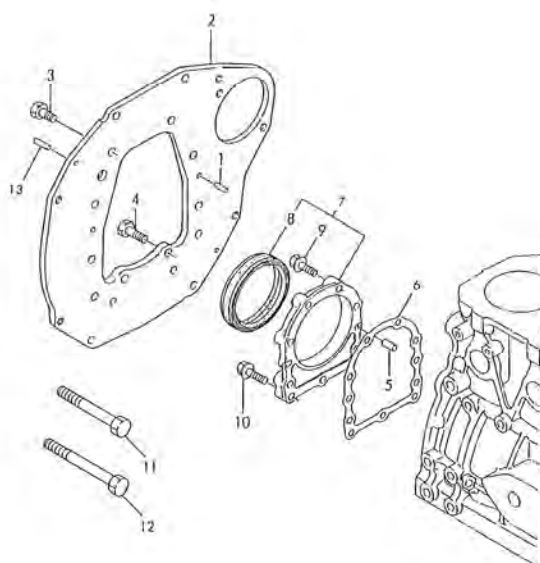
Fig. 3 マウンティングフランジ MOUNTING FLANGE
