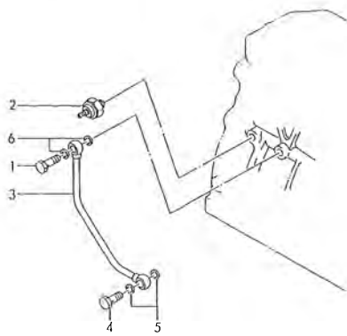
Fig. 12 LOパイプ LUB. OIL LINE
