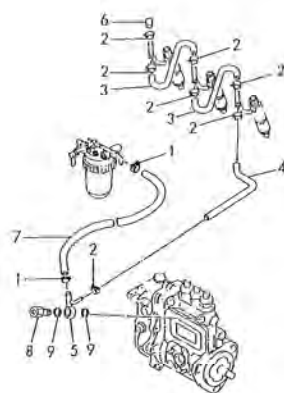
Fig. 18 FO モドシバイブ FUEL RETURN LINE
