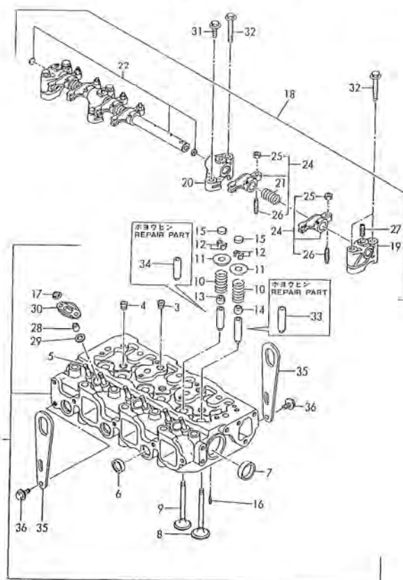
Fig. 6 シリンダヘッド CYLINDER HEAD
