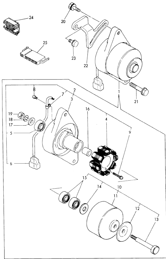
Fig. 15 GENERATOR
