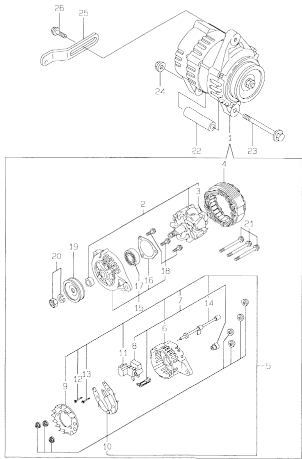
Fig.17. GENERATOR
