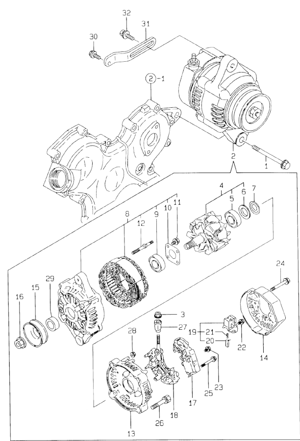
Fig.15. GENERATOR
