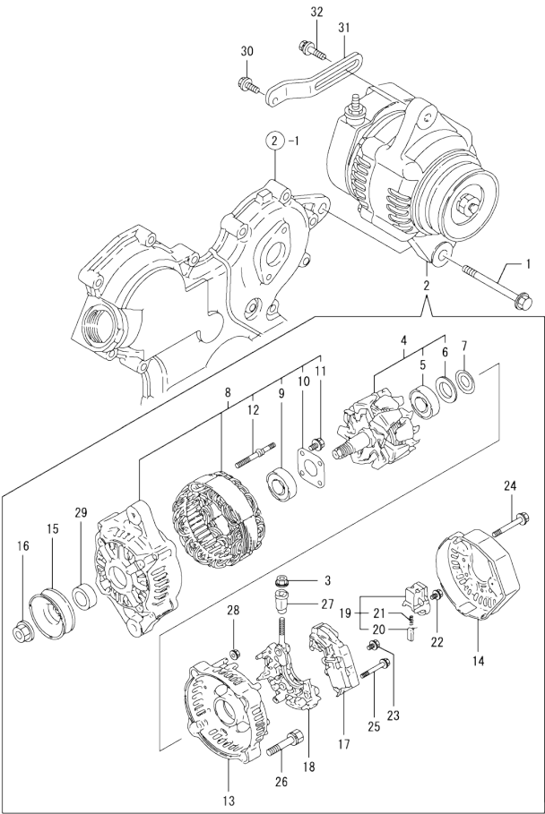
Fig.16. GENERATOR
