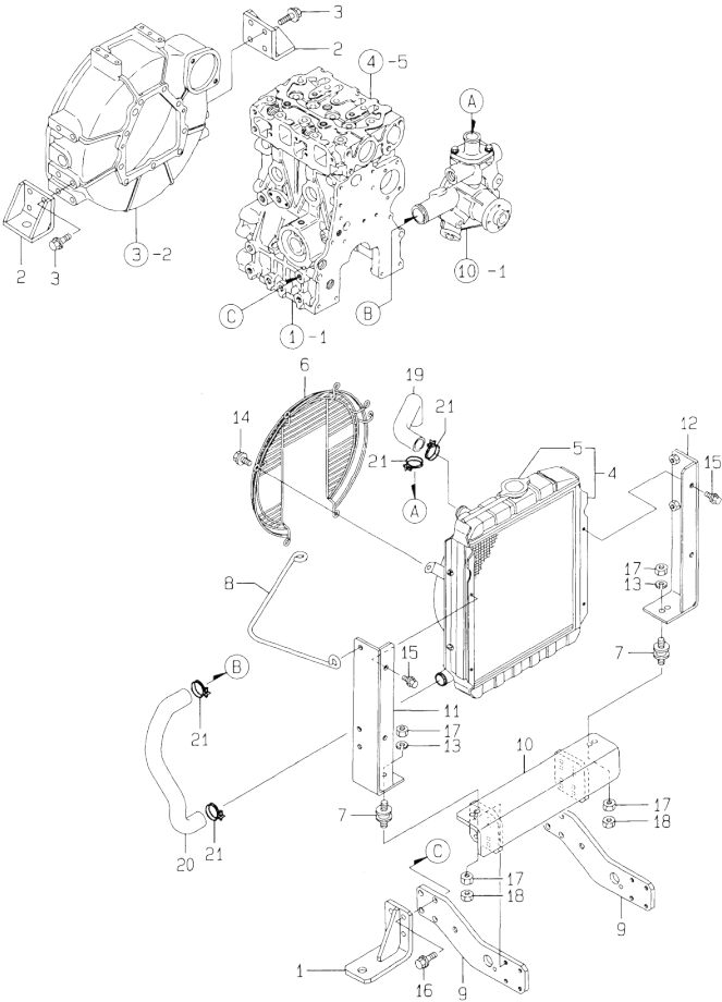
Fig.11. RADIATOR
