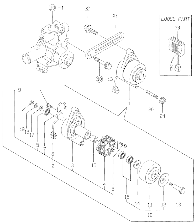
Fig.16. GENERATOR
