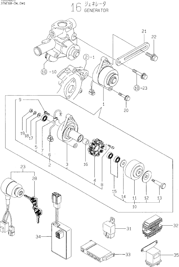
Fig.16. GENERATOR
