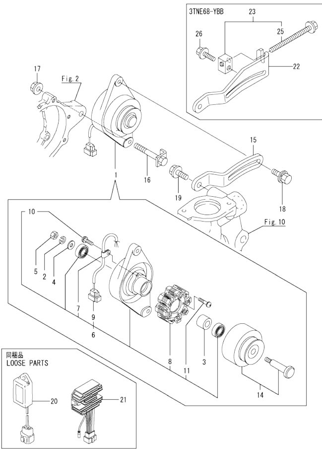
Fig.15. GENERATOR
