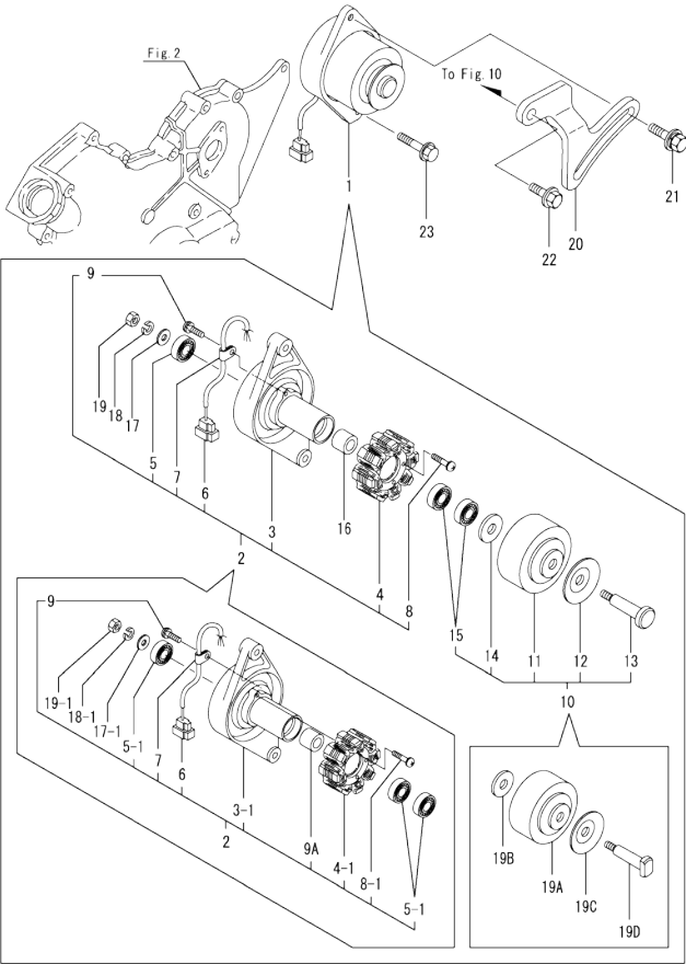
Fig.16. GENERATOR
