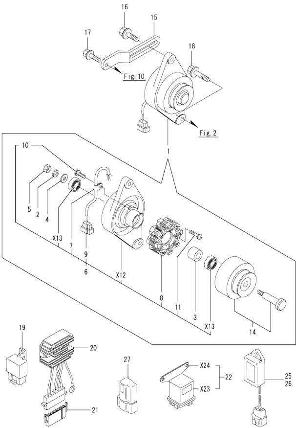
Fig.16. GENERATOR
