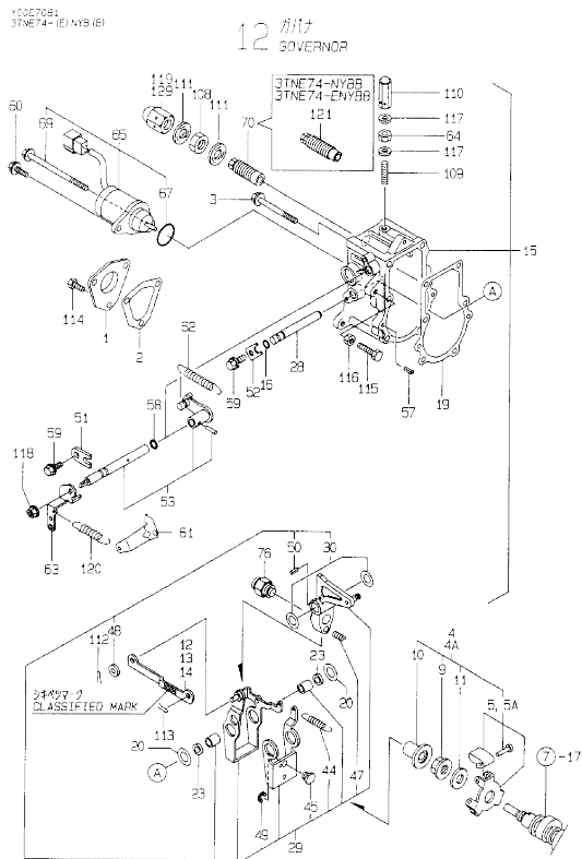
OCD10-M70801 3TNE74-(E)NYB(B) Fig.12. GOVERNOR
