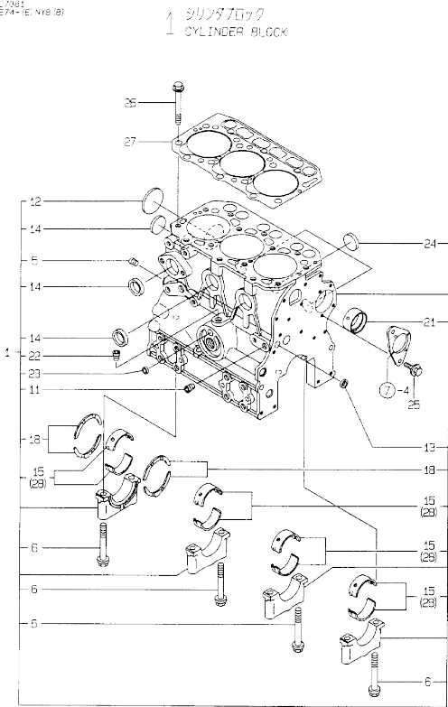
OCD10-M70801 3TNE74-(E)NYB(B) Fig.1. CYLINDER BLOCK
