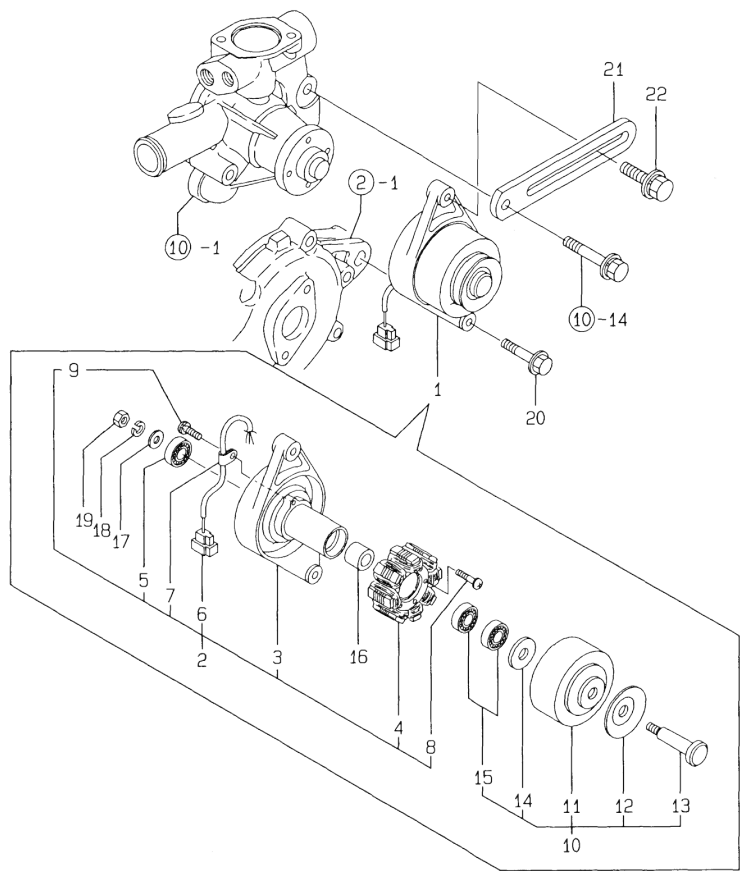
Fig.16. GENERATOR
