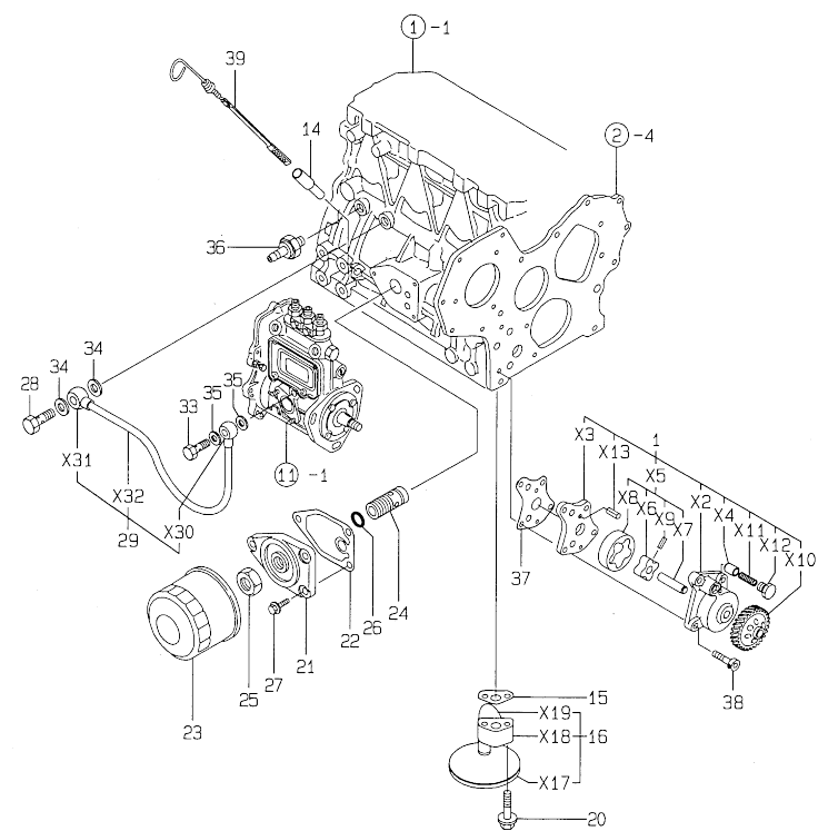
0CV10-M41200 3TNE78A-ADCL Fig.9. LUB.OIL SYSTEM
