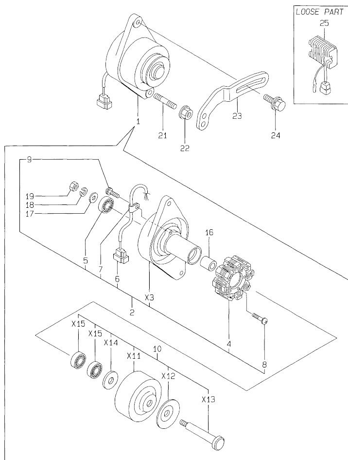
16. GENERATOR
