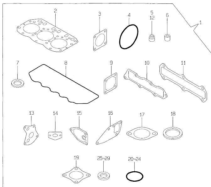
17. GASKET SET
