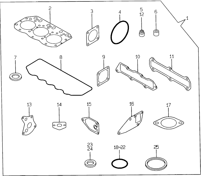
Fig.16. GASKET SET
