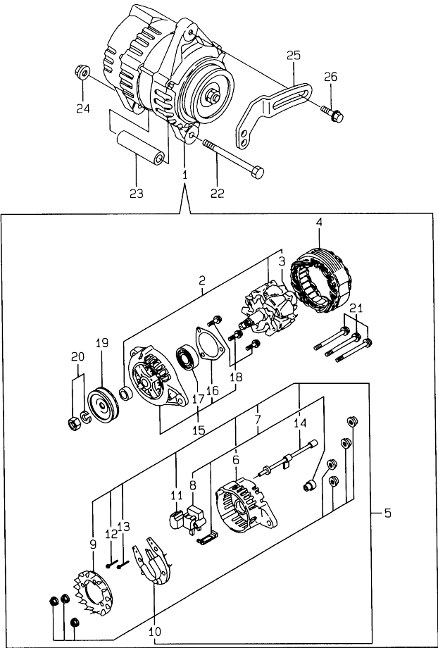
Fig.15. GENERATOR
