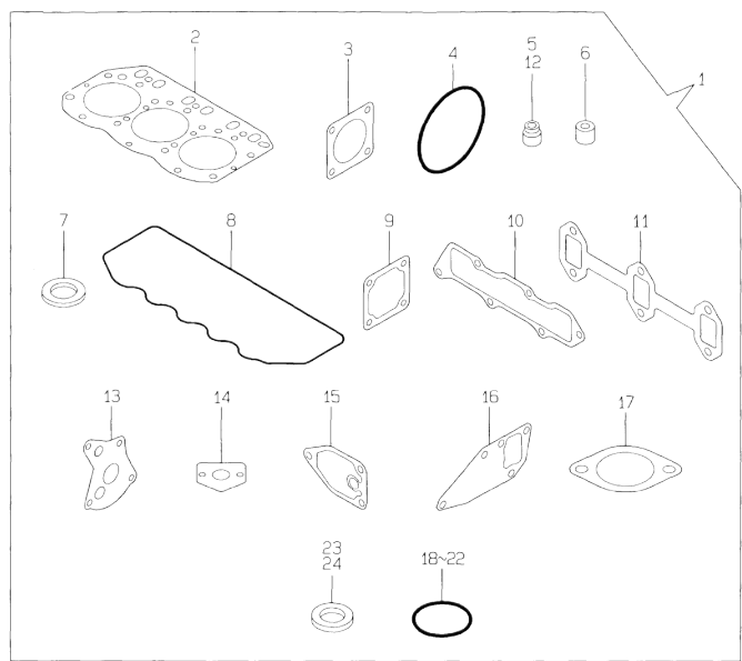
Fig.15. GASKET SET
